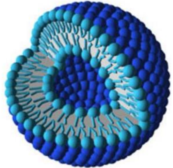
Холестери
