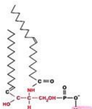
Сфингомиелин
