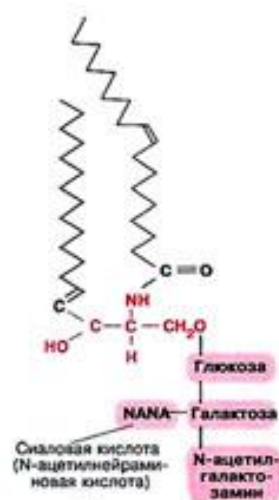
Ганглиозид
